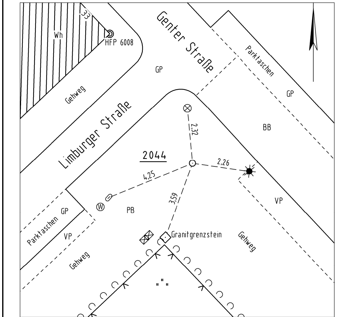
Einmesssskizze
