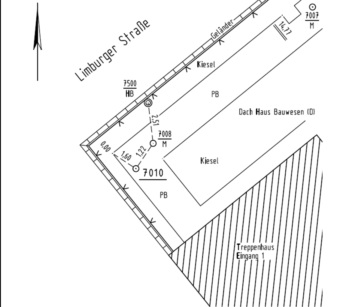
Einmessskizze
